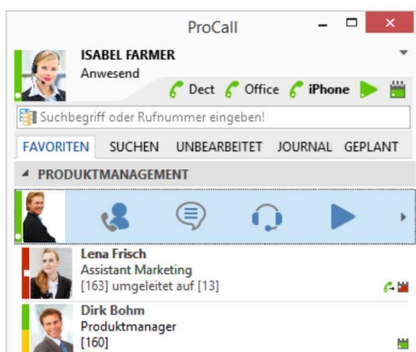
ProCall Hauptfenster
