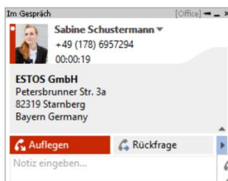
ProCall Gesprächsfenster
